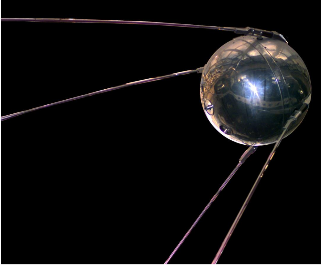
1- satélite Sputnik
