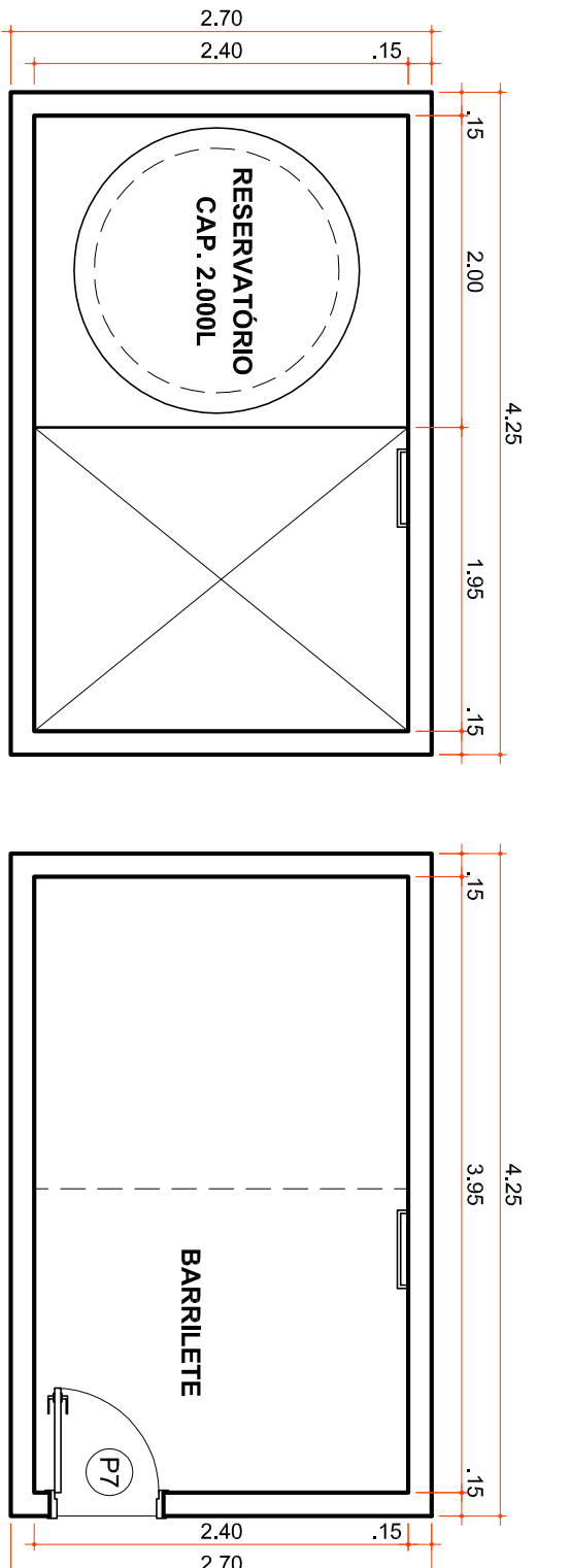
RESERVATÓRIO Área: 17,28 m² Escala: 1:50
