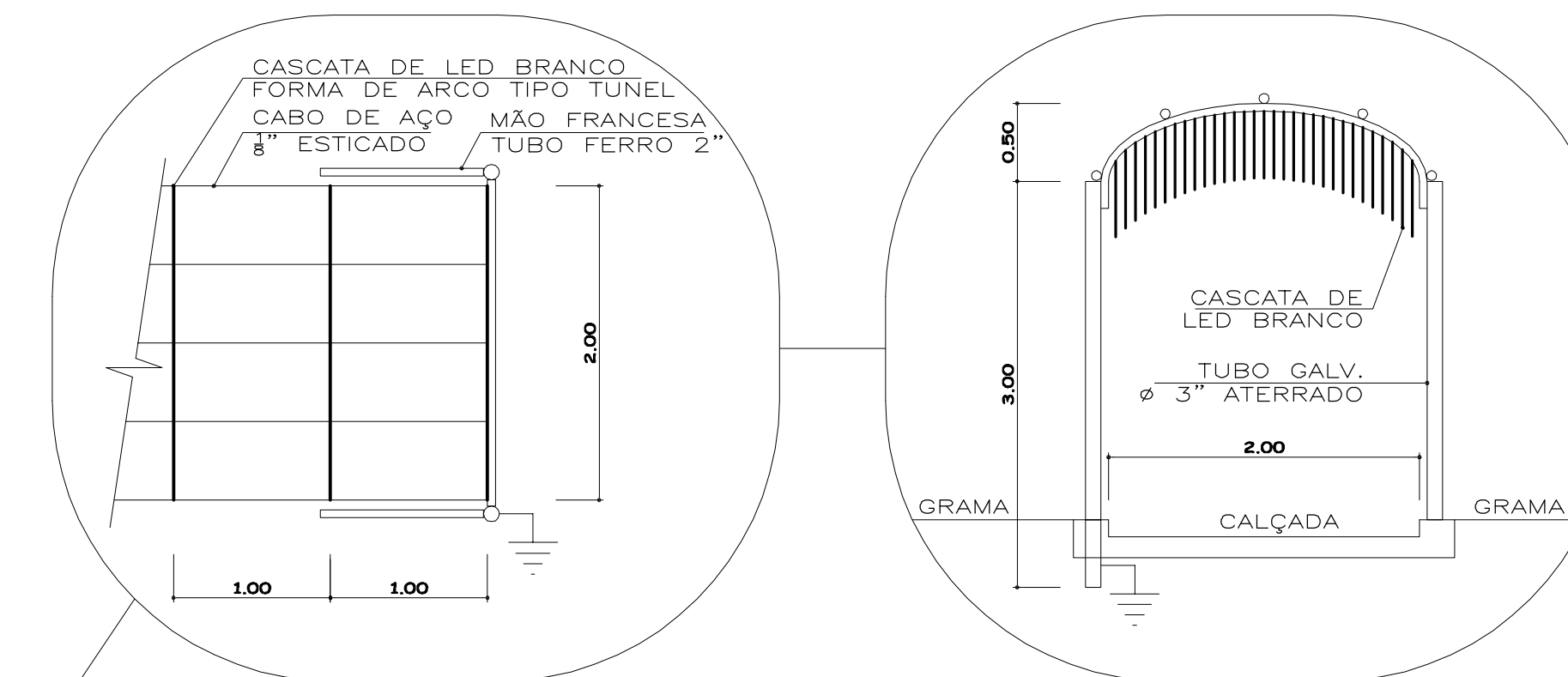
DETALHE TUNEL SEM ESCALA
