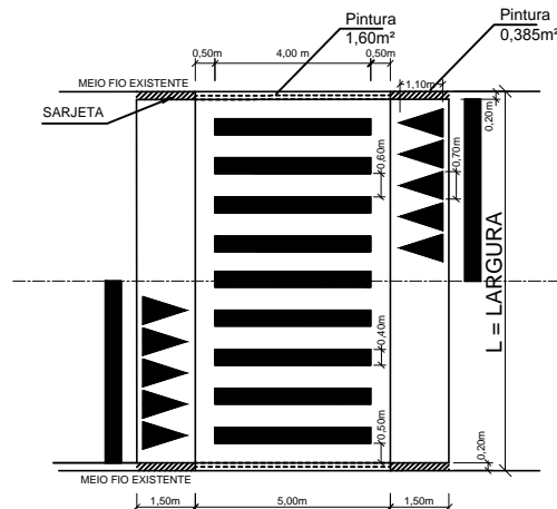
DETALHE 2 SEM / ESC.
