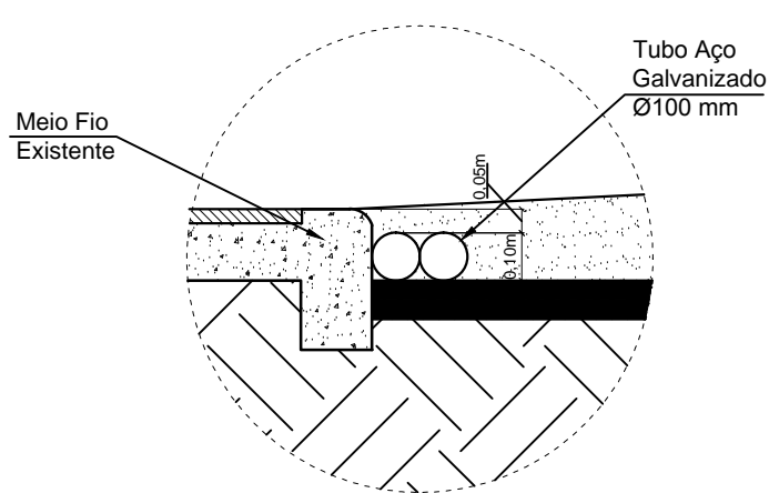
DETALHE 01 SEM ESCALA
