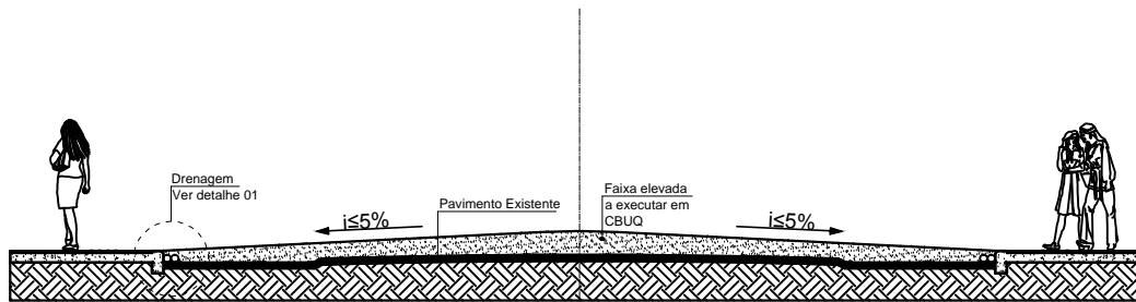
Faixa Elevada - Perfil Longitudinal
